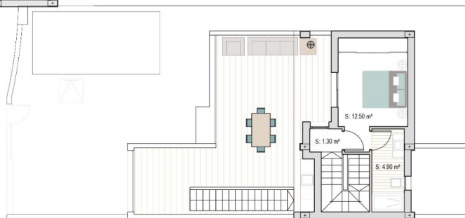
Planta primera
